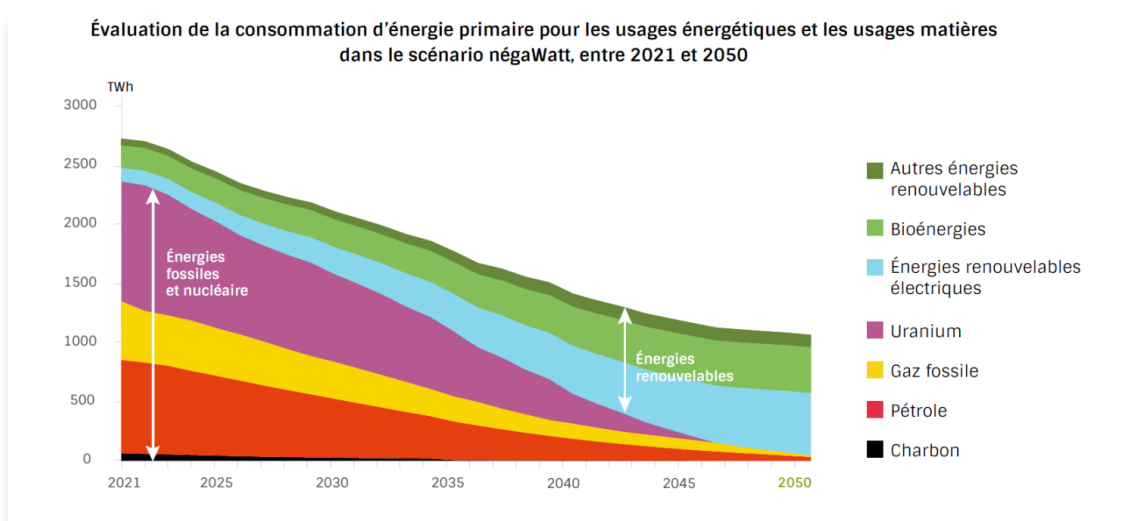
L'évolution des sources d'énergie dans le scénario négaWatt. © Négawatt
